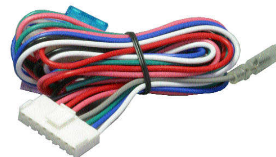
LOCK/UNLOCK・ドアトリガー・電源入力ハーネス
