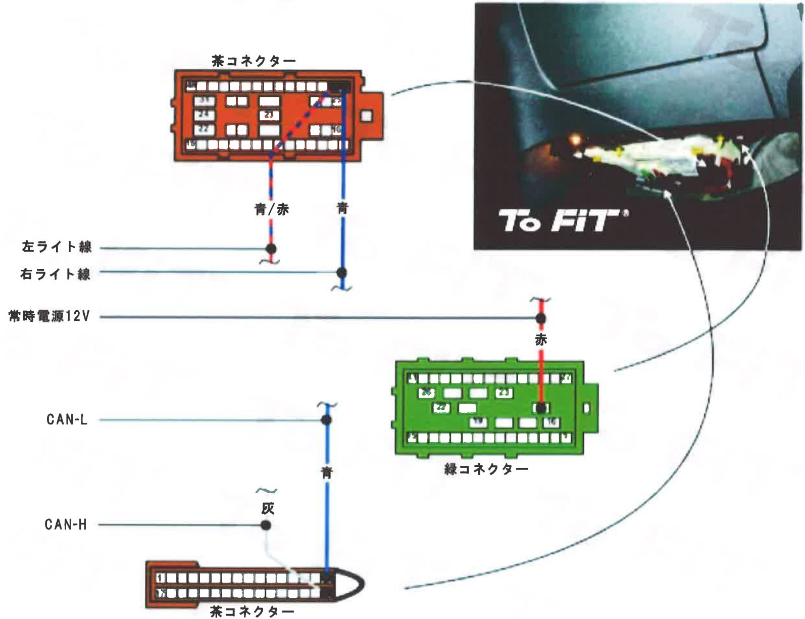
CAN線は2本より線になっています
